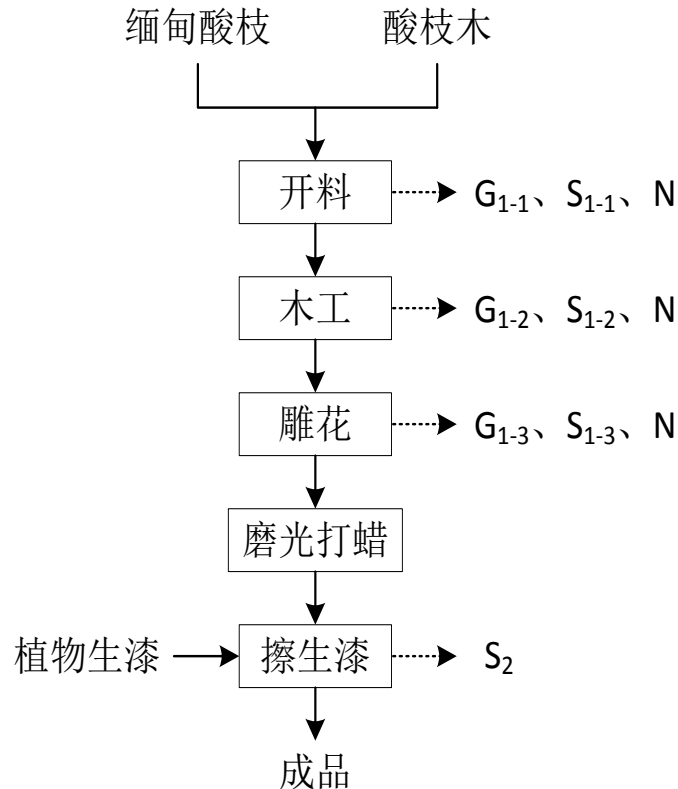
图 5-1 红木家具生产工艺流程及产污环节图
