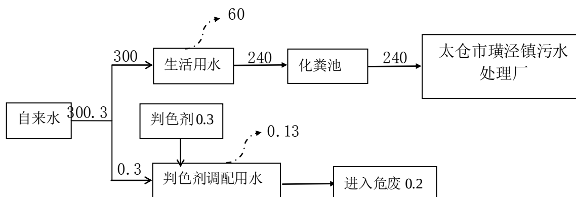
图 5-2 本项目水平衡图 (t/a)
