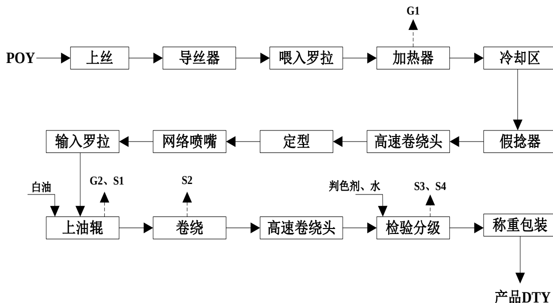
图 5-1 涤纶加弹丝生产工艺流程及产污节点图
