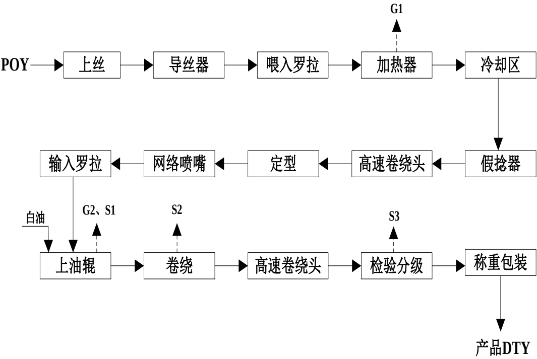
图 5-1 涤纶加弹丝生产工艺流程及产污节点图
