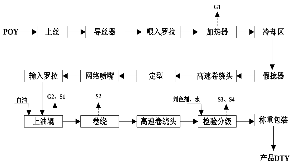
图 5-1 涤纶 DTY 加弹丝生产工艺流程及产污节点图
