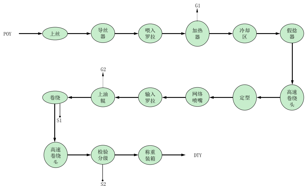
图 5-1 DTY 生产工艺流程
