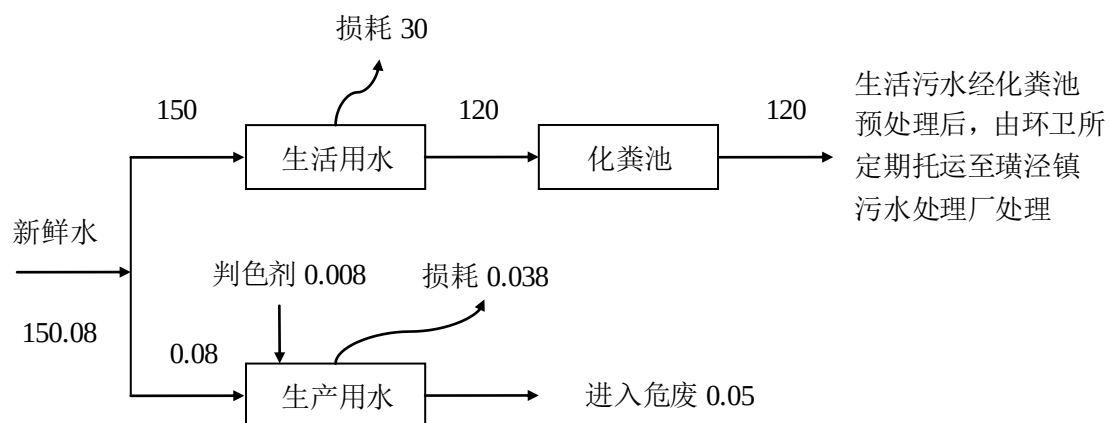
图 1-2 原有项目水平衡图 (t/a)
