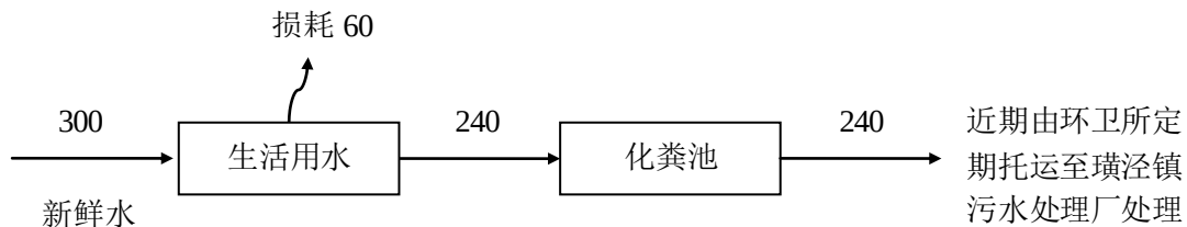
图 5-2 本项目水平衡图 (t/a)
