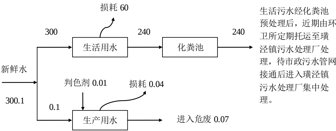
图 5-2 扩建项目水平衡图 (t/a)
