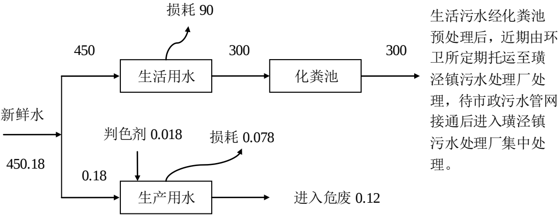
图 5-3 扩建后全厂水平衡图 (t/a)
