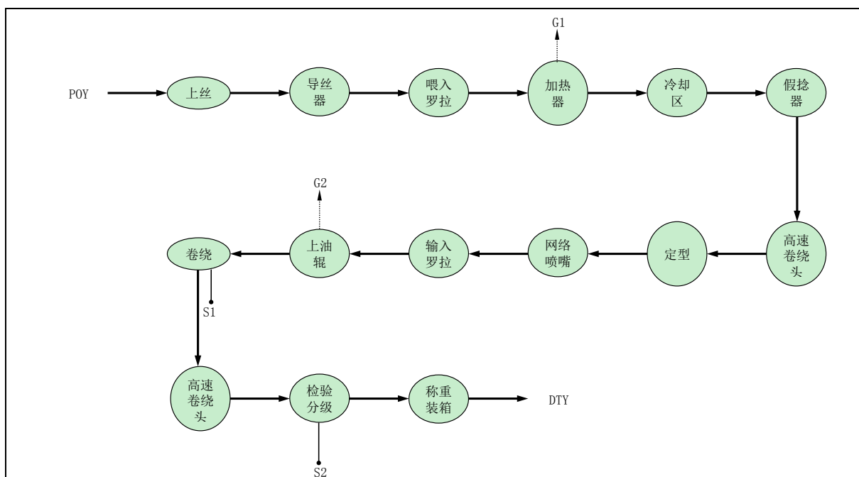
图 1-1 涤纶加弹丝生产工艺流程及产污环节图
