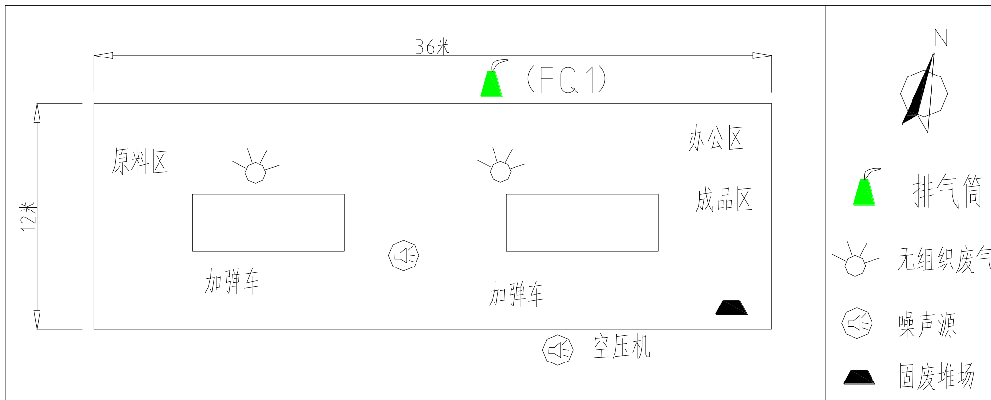
附图 3 厂区平面布置图
