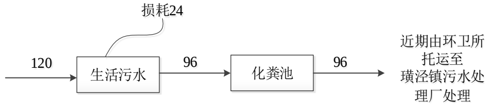
图 5-2 本项目水平衡图 (t/a)
