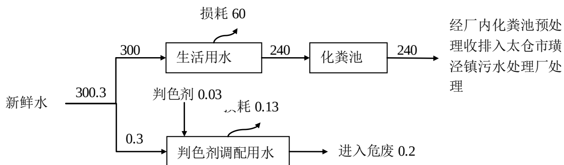
图 5-2 本项目水平衡图 (t/a)
