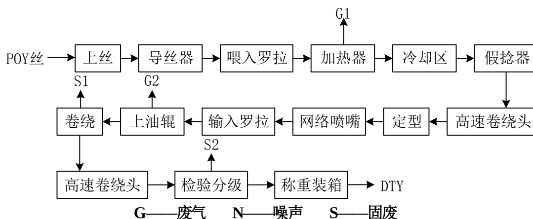
图 5-1 涤纶 DTY 加弹丝生产工艺流程及产污节点图
