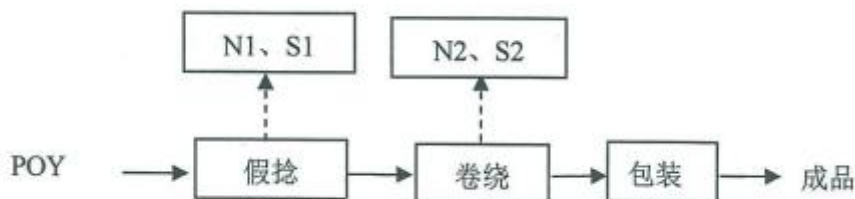
图 1-1 加弹丝生产工艺流程及产污环节图
