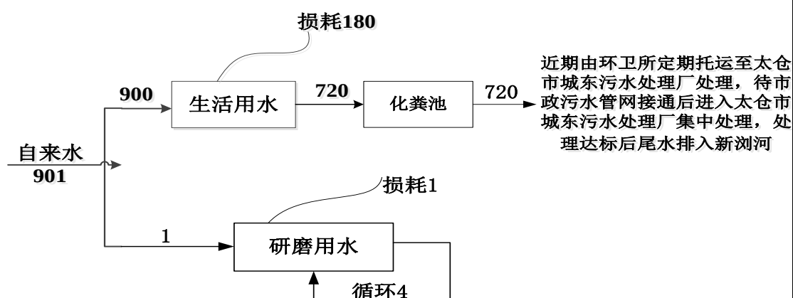
图 5-2 本项目水平衡图 单位： t/a
