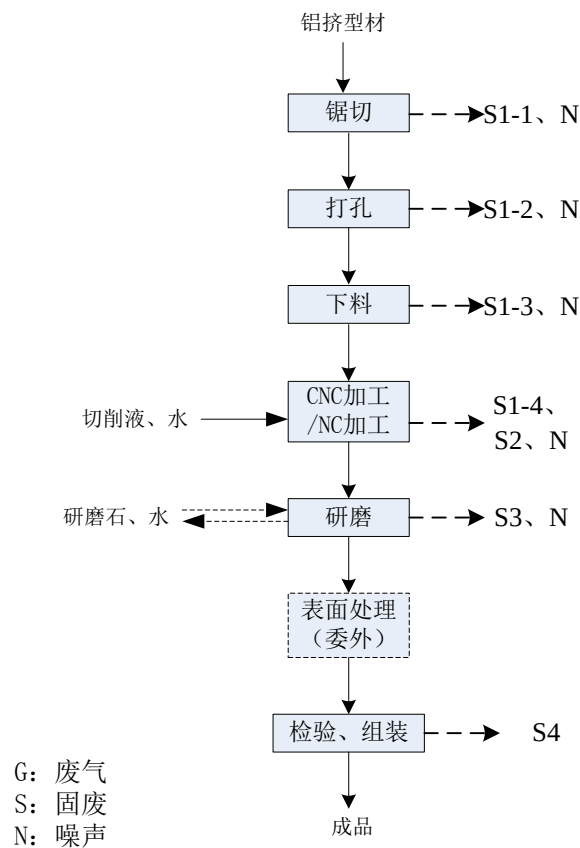
图 5-1 机械零部件生产工艺及产污环节图
