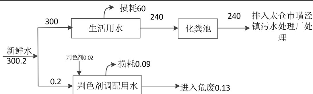
图 5-2 扩建项目水平衡图 (t/a)
