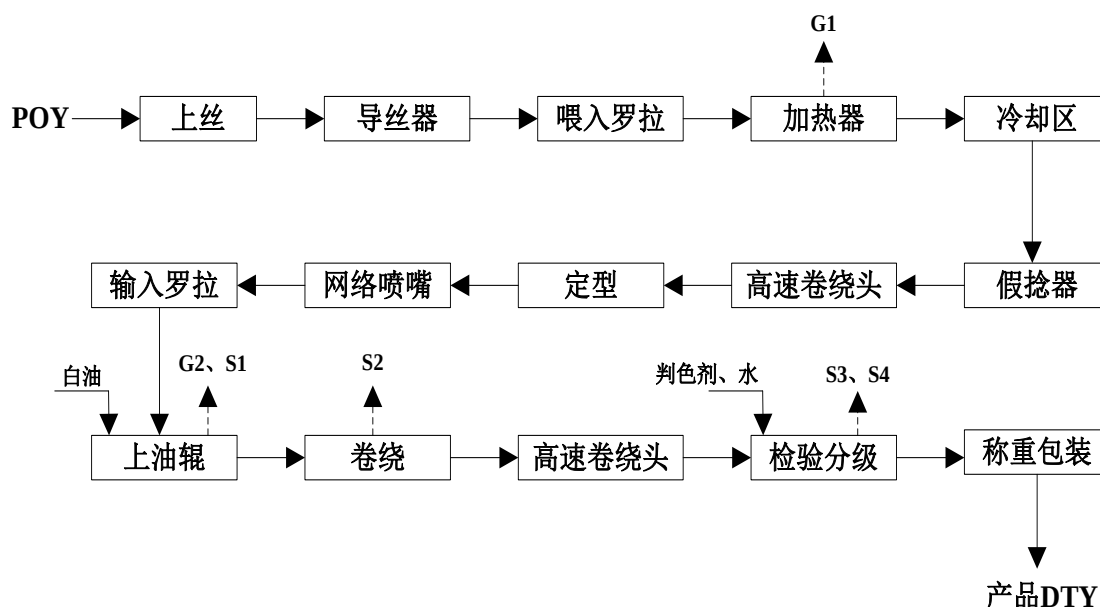
图 5-1 DTY 生产工艺流程
