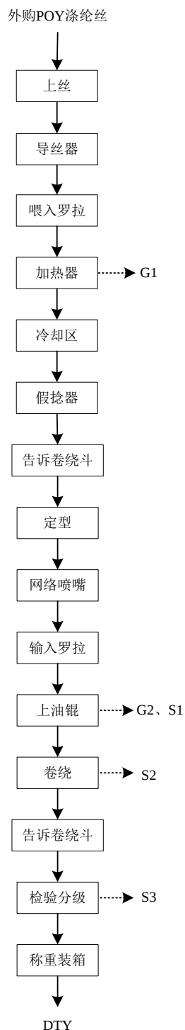
图 1-1 加弹丝生产工艺流程及产污环节图
