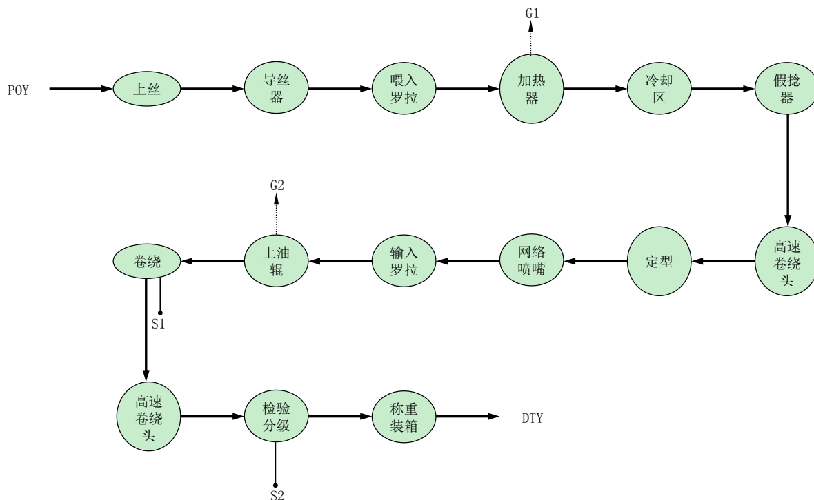
图 1-1 加弹丝生产工艺流程及产污环节图
