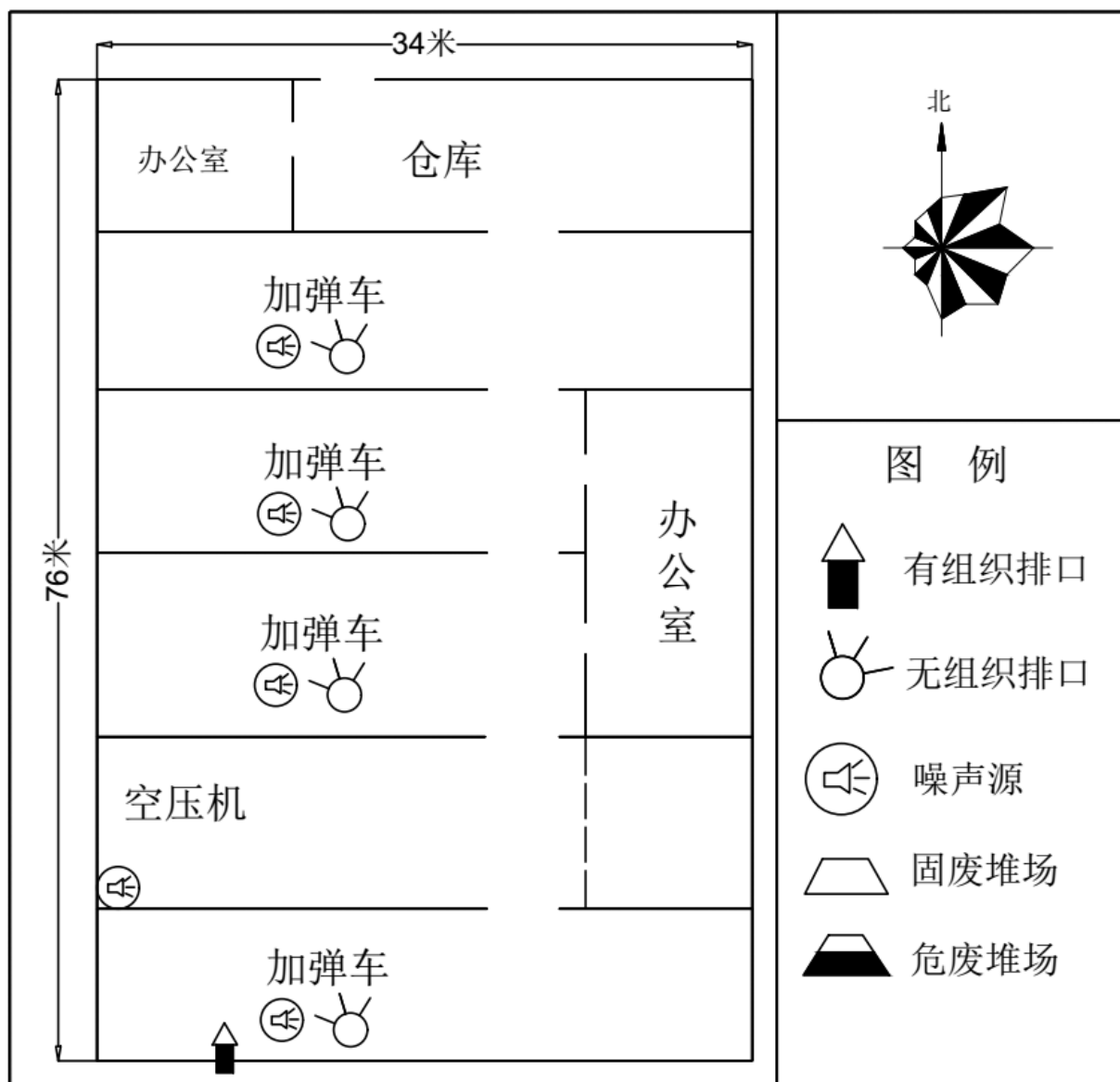
附图 3 项目平面布置图
