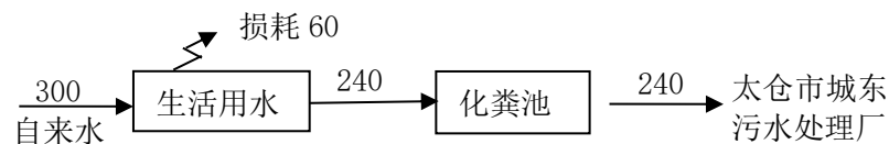
图 5 建设项目全厂用排水平衡图 （单位 t/a）
