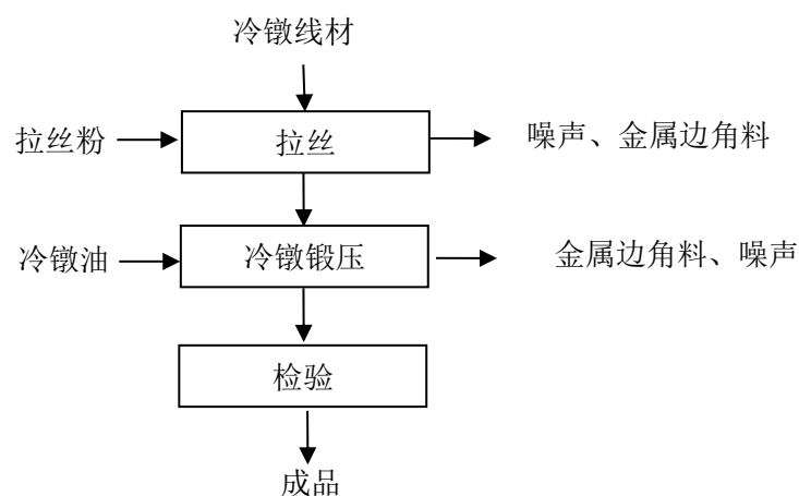
图 4 建设项目金属制品生产工艺流程图
