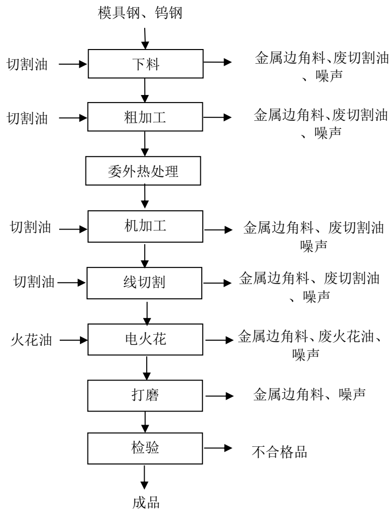
图 3 建设项目模具生产工艺流程图
