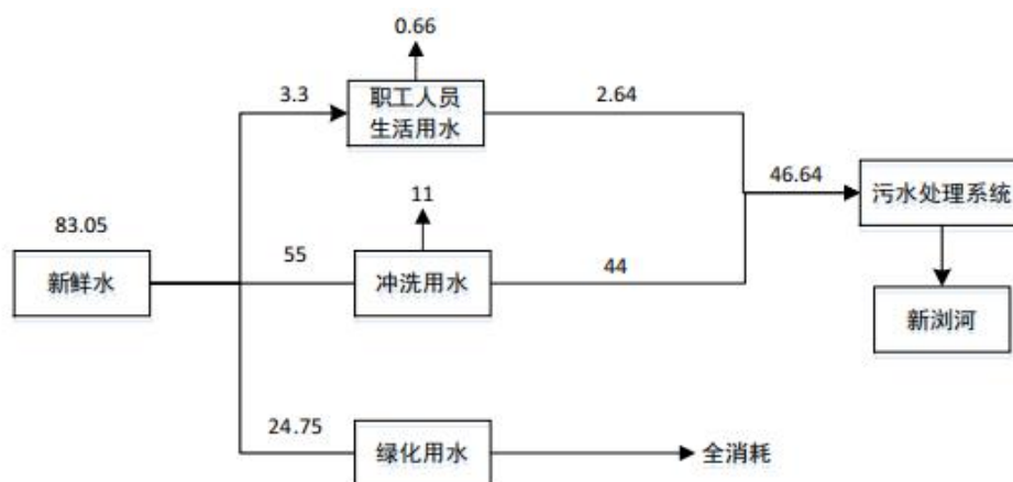
图 4-1 项目厂区内水平衡图 (m³/a)
